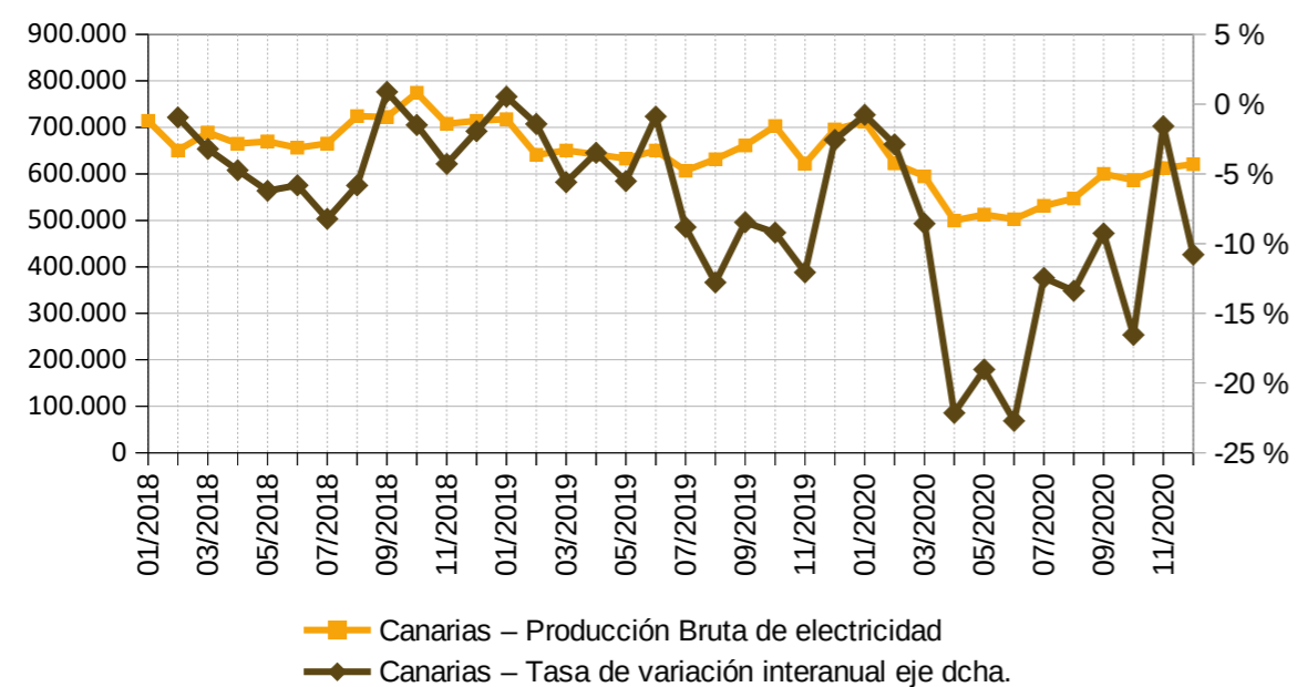
GRÁFICO 4.14. EVOLUCIÓN DE LA PRODUCCIÓN BRUTA DE ELECTRICIDAD EN CANARIAS (Mwh y tasa de variación interanual). 2018-2020
