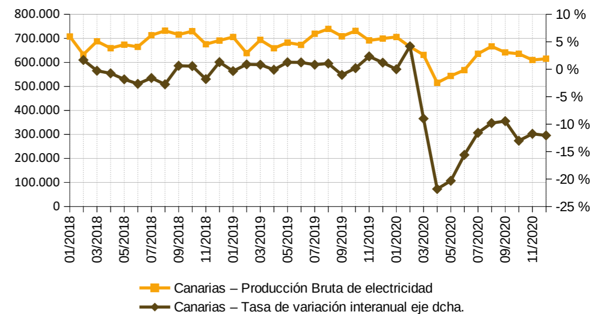
GRÁFICO 4.15. EVOLUCIÓN DE LA ENERGÍA ELÉCTRICA DISPONIBLE PARA CONSUMO FINAL EN CANARIAS (Mwh y tasa de variación interanual). 2018-2020
